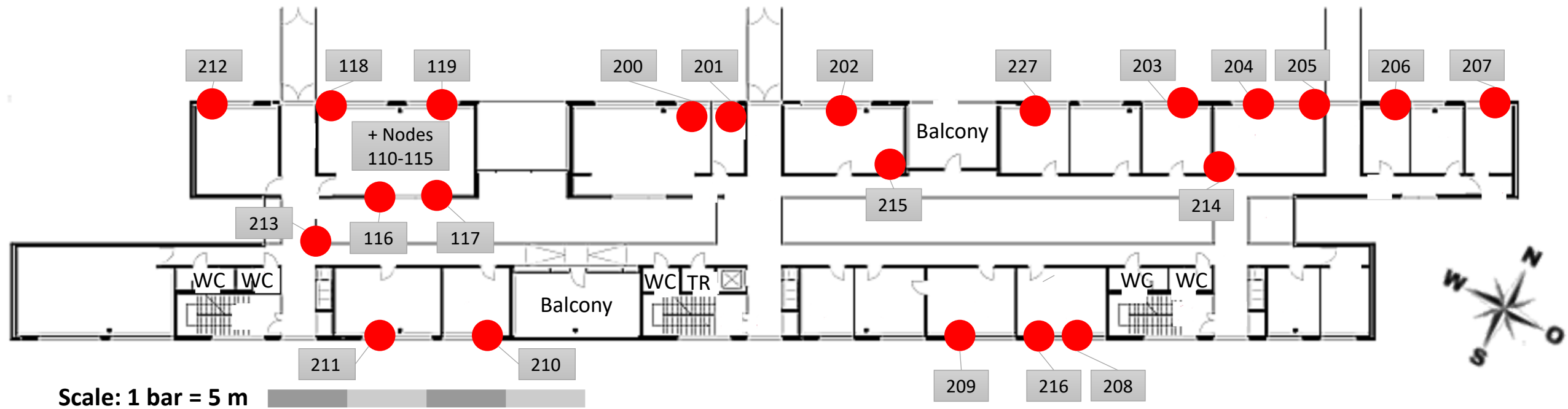
Inffeldgasse 16, 1. OG
